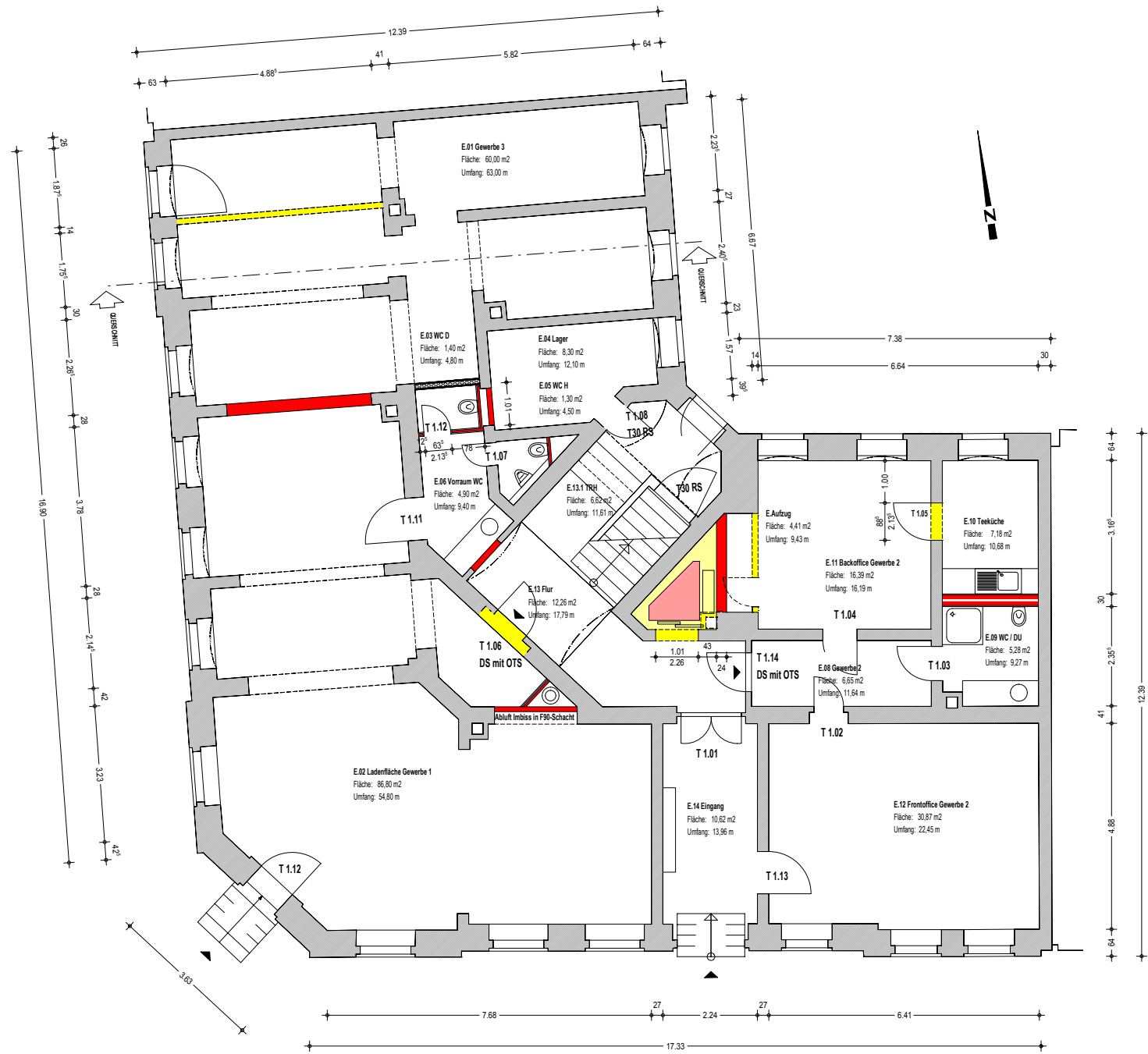
GRUNDRISS ERDGESCHOSS LOHRSTRASSE 2014_02_09
