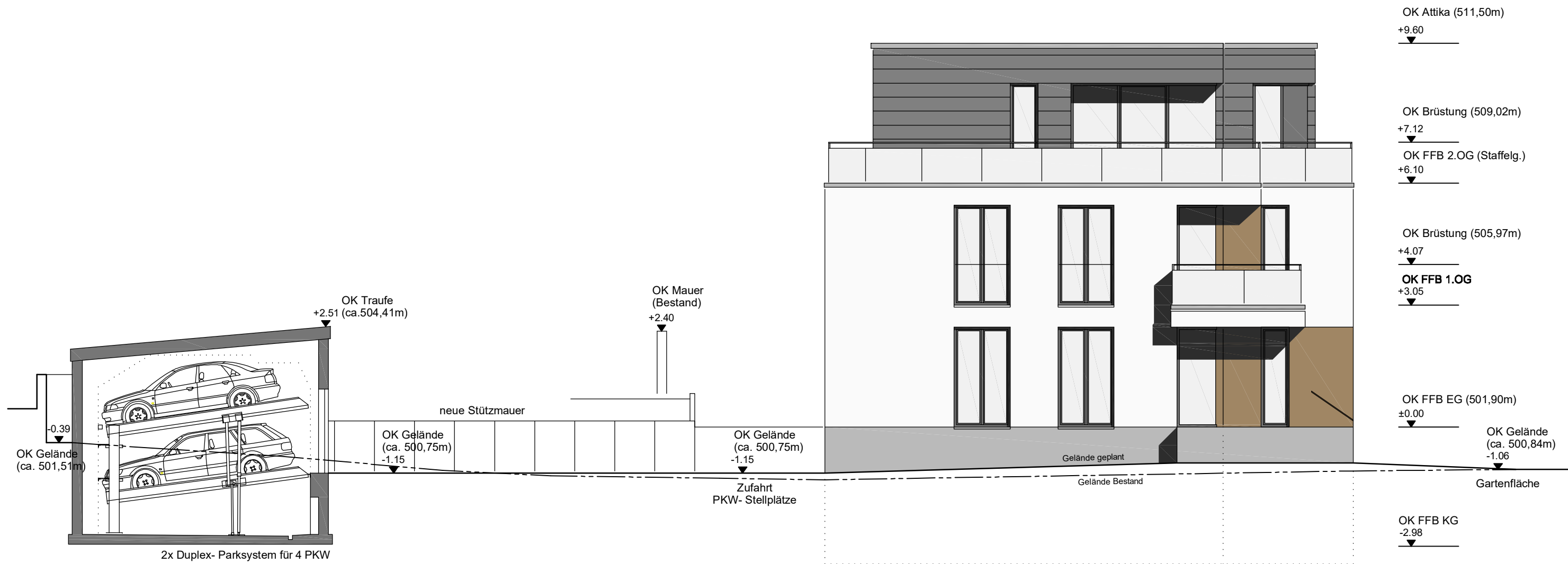
ANSICHT WEST
