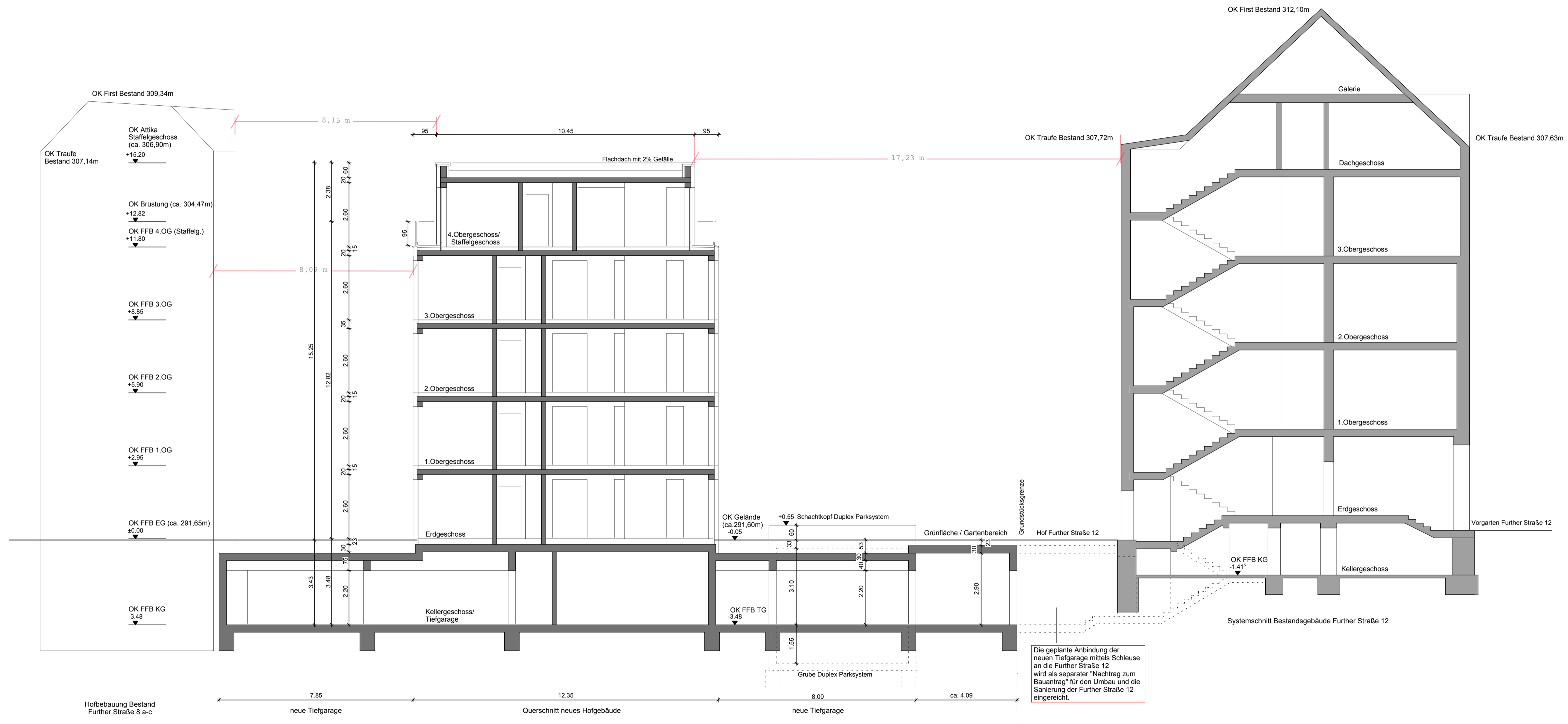
SCHNITT A - A
